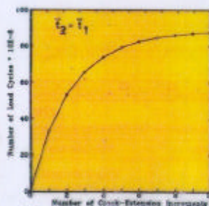
Fatigue life diagram
